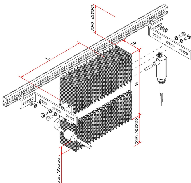
Изображение 3: Пример монтажа VARITHERM в вертикальном положении с TAE или TS с соблюдением минимального расстояния
